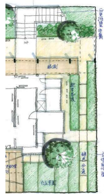
21 棟展示保育社區中心平面圖 SCALE: 1/60
